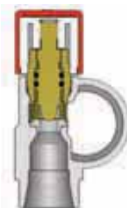
Рис. 20. Запорно-балансировочный коллектор
