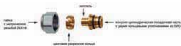
Рис. 36. Концовка FAR для пластиковых труб
